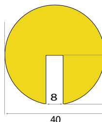
Typ B: Profil för montering på kanter (rund utan tape)
