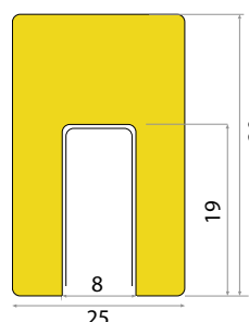
Typ G: Profil för montering på kanter (med tape)
