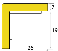
Typ E: Profil för montering på kanter (platt med tape)
