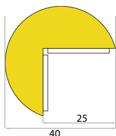
Typ A: Profil för montering på kanter (rund med tape)
