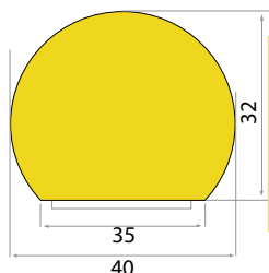
Typ C: Profil för montering på platt underlag (rund med tape)
